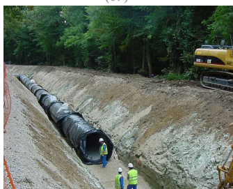
SDEA BETON Ø 2 200 EP - LE POUZIN (07)
